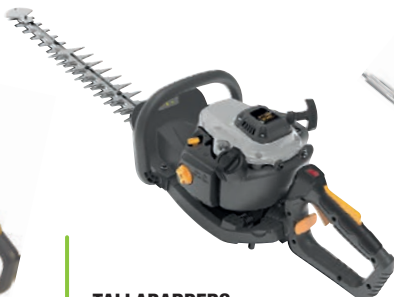
TALLABARDERS A GASOLINA 9704381 Potència 0,65 kW. Fulla doble acció de 700 mm amb protector metàl·lic 56 cm de tall, manillar giratori de 180°, ample de tall 27 mm.
